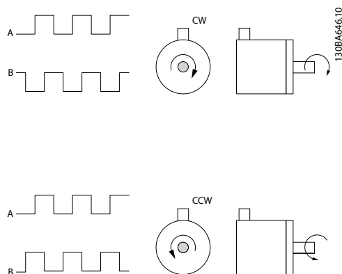
Рисунок 6.3 Инкрементальный энкодер 24 В. Макс. длина кабеля — 5 м.
