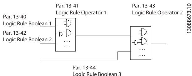
Рисунок 2.37 Правила логики
