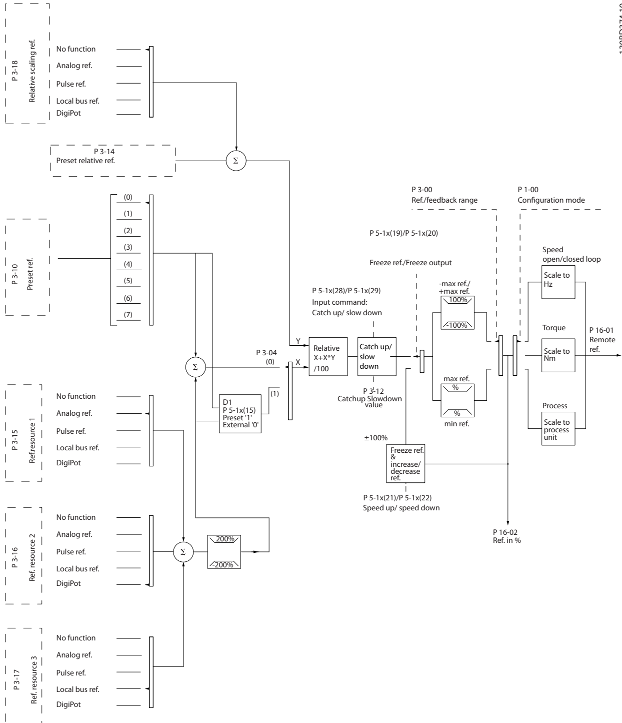
Рисунок 2.14 Дистанционное задание
