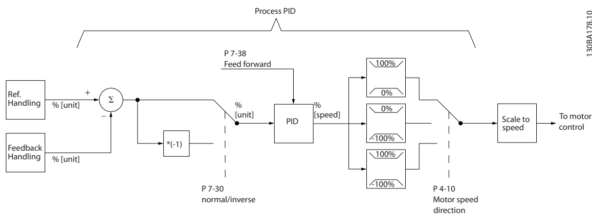
Рисунок 2.23 Схема ПИД-регулятора процесса
