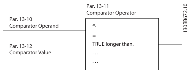
Рисунок 2.36 Компараторы
