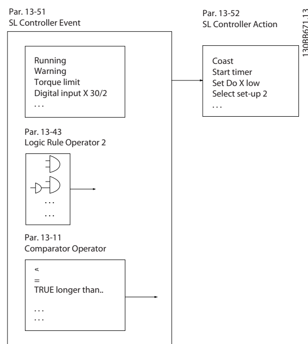
Рисунок 2.34 Связанное действие
